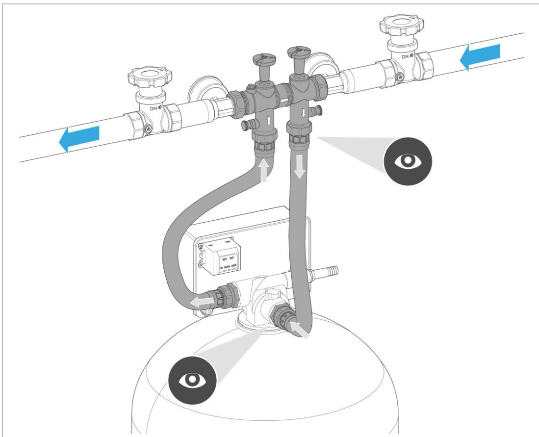
Kiesfilter DN 40 mit Anschluss-Set 1½"
