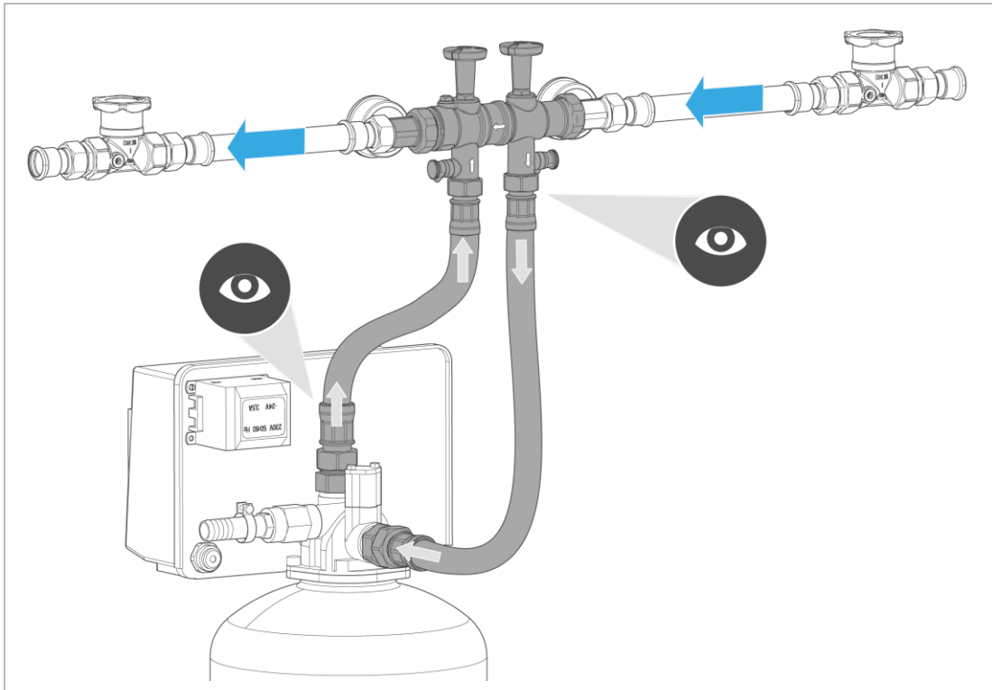
Kiesfilter DN 40 mit Anschluss-Set 1½"
