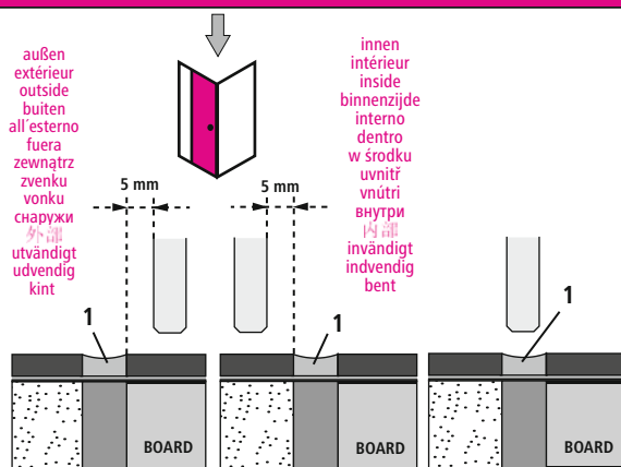
2 Versiegelung / Scellement / Sealing / Siliconen-kitnaad / Sigillatura Sellado / Uszczelnienie zewnętrzne / Uzavirací náter / Tesniaca hmota Герметик / 密封胶 / Försigling / Försigling / Elzárás
