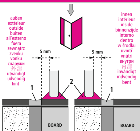
1 Wartungsfuge / Joint de maintenance / Maintenance joint / Voegnaad / Fughe di manutenzione Junta de mantenimiento / Spoina wymagająca konserwacji / Spära pro údržbu / Servisná medzera Технологический шов / 维护缝 / Underhållstog / Vedligeholdelsesfuge / szilikon fuga
