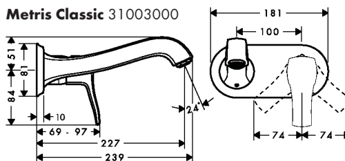
Metris 31085000 / 31251000
