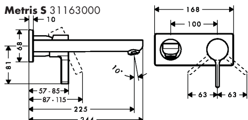
Metris S 31163000
