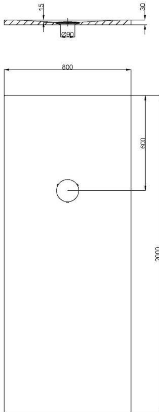
Duschwannen Nias 2000x800 Rechteck 4560xA ungeschnitten
