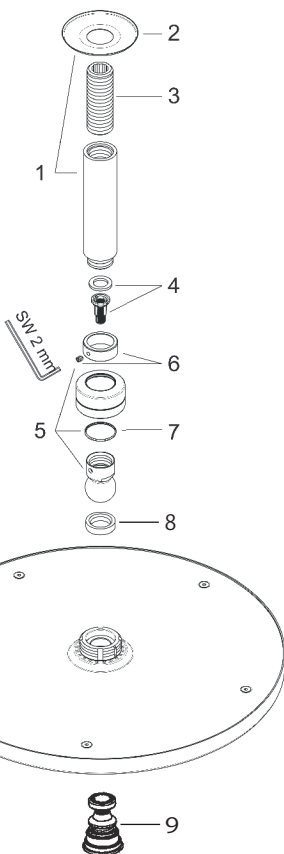
製品分解図
