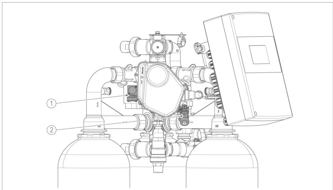
Bezeichnung 1 Injektor
