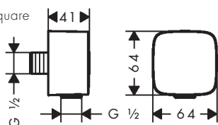
AXOR Fixfit square 36732XX0
