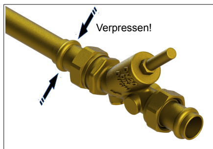
Montageschritt 4
